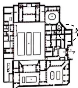
تصویر ۲۲: نقشه اشکوب اول عمارت مشیر دیوان در شهر سنندج (آرشیو میراث فرهنگی استان کردستان)
